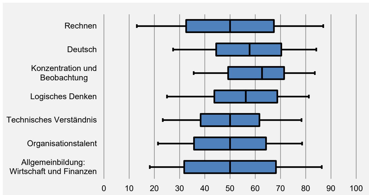
Grafik 3 Boxplot*
